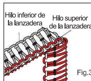
Baja tensión del hilo de la lanzadera superior o alta tensión del hilo de la lanzadera inferior.
