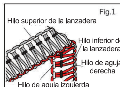
Hilo de aguja correcto.
