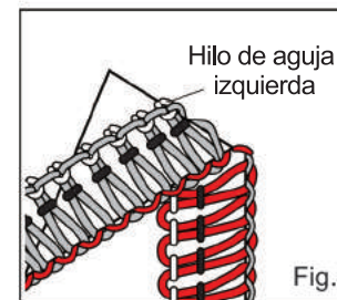
Baja tensión del hilo de la aguja izquierda.
